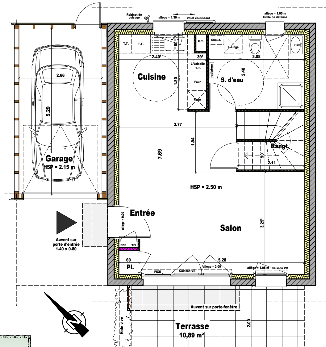
Lot -05- (P.S.L.A.) Plan: Rez de chaussée
